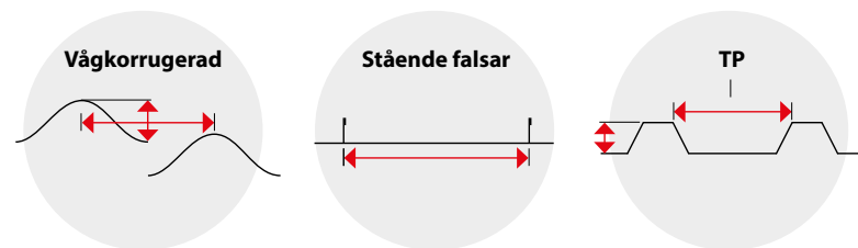
Exempel på olika plåtprofiler och hur du mäter.
